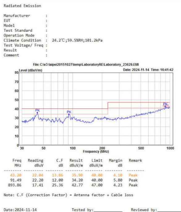
图 4-6 RE 测试垂直方向
