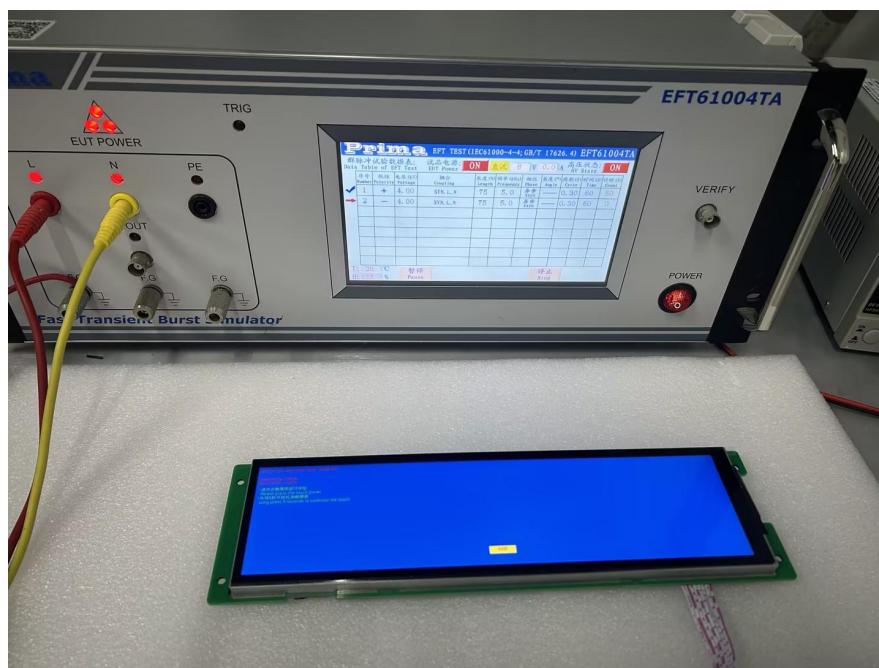
图 4-3 EFT 测试图
